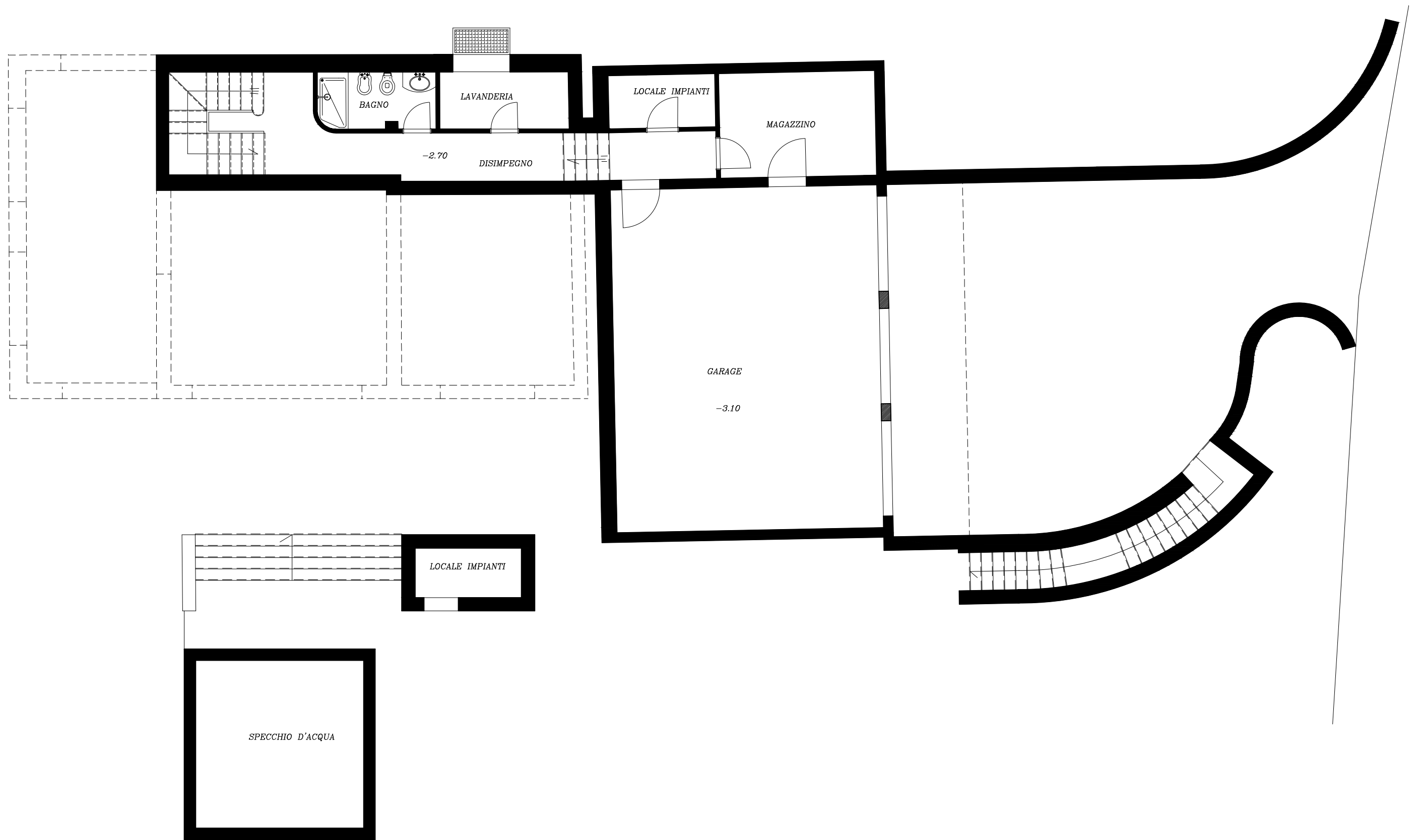
PIANTA PIANO INTERRATO
